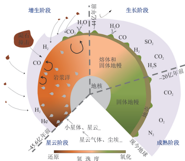
图2 行星起源、挥发分和地球演化
