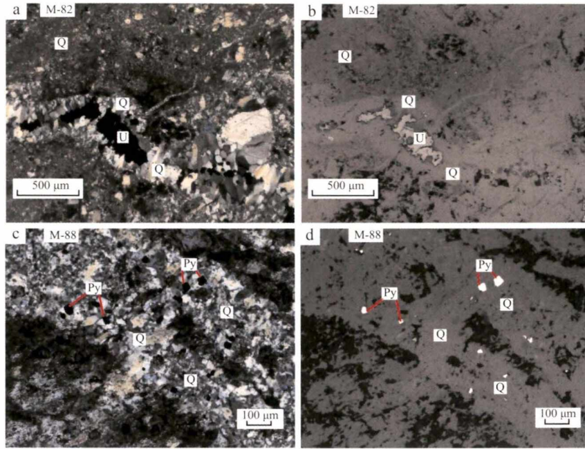
图4 硅质脉型铀矿石(M-88)显微特征
