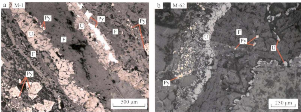
图3 萤石型铀矿石(M-62)显微特征
