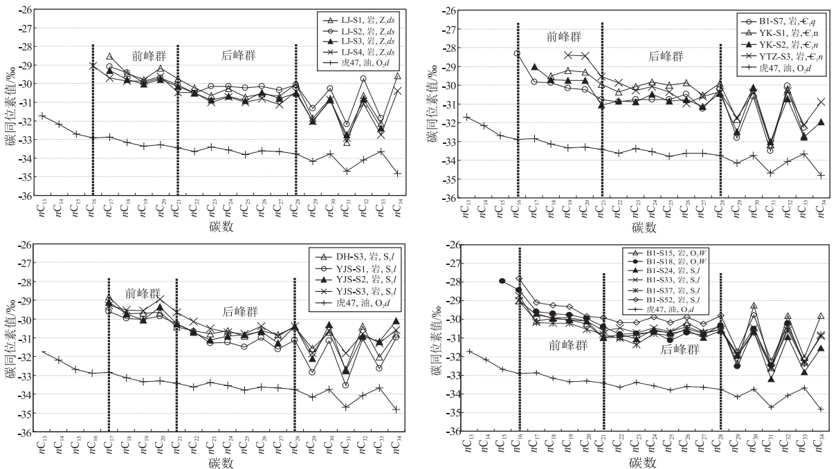
图 5 黔北和黔南拗陷不同层位烃源岩和虎 47 井原油中正构烷烃单体烃碳同位素组成对比
