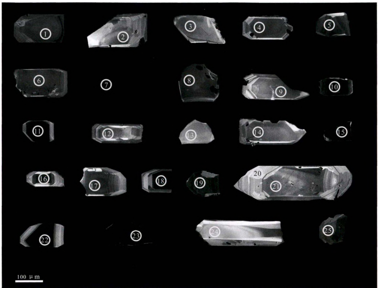
图 6 秦皇岛石门寨孙家梁组流纹岩锆石阴极发光图像(CL)
