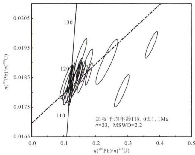
图 7 秦皇岛石门寨孙家梁组流纹岩 LA-ICP-MS 锆石 U-Pb 谐和图
