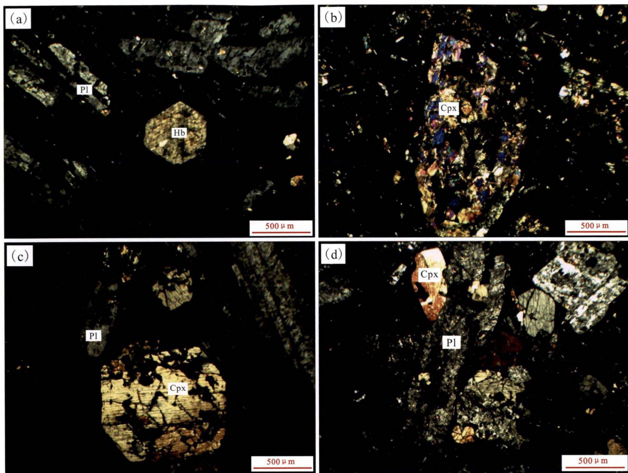
图3 秦皇岛石门寨蓝旗组代表性火山岩显微照片
