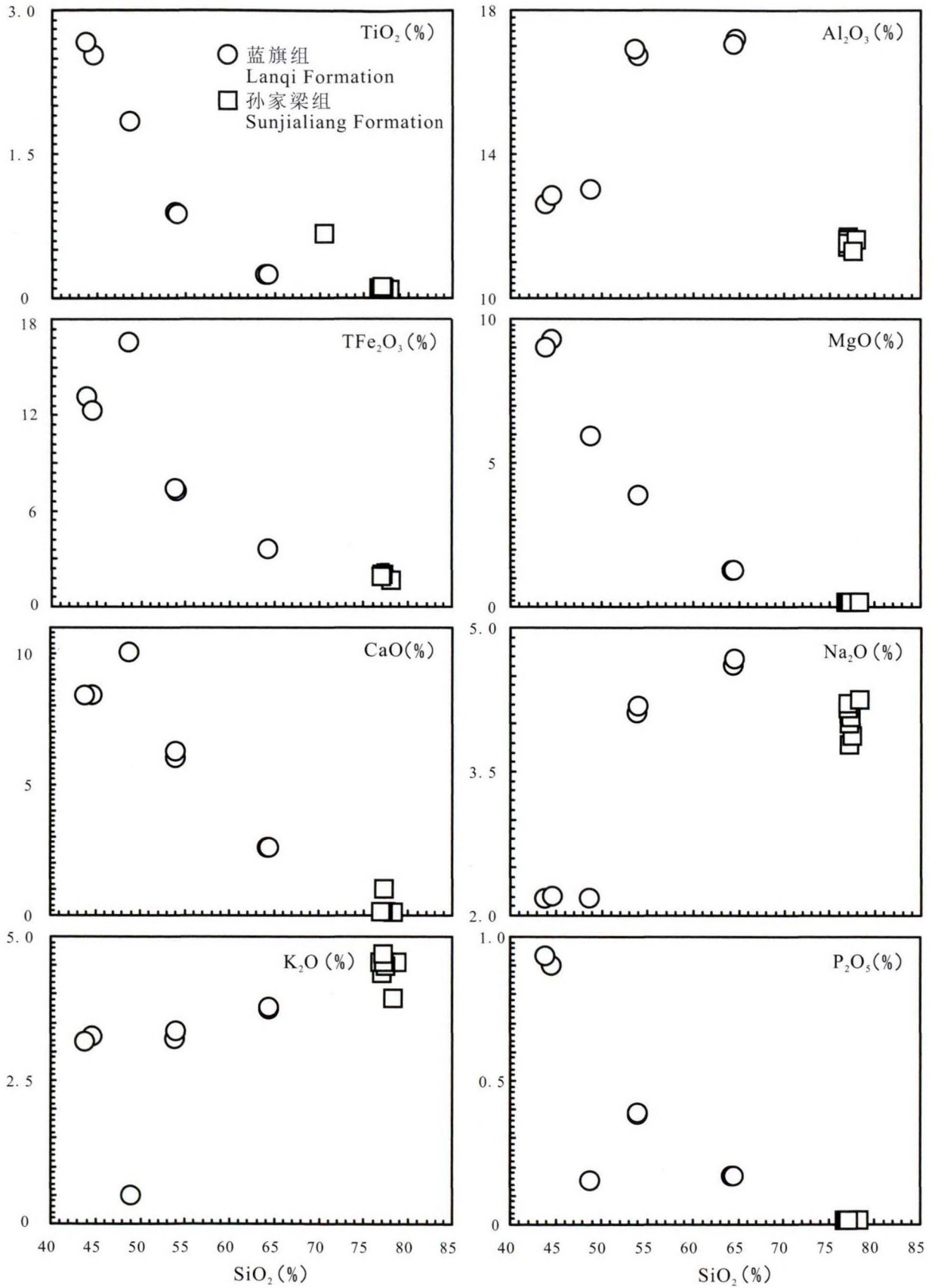
图5 秦皇岛石门寨蓝旗组和孙家梁组火山岩岩石化学成分哈克图解
