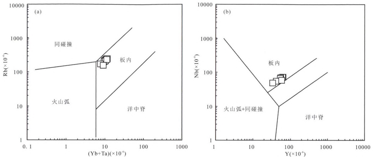
图 11 秦皇岛石门寨孙家梁组火山岩 (Yb+Ta)—Rb(a) 和 Y—Nb(b) 构造环境判别图解(据 Pearce et al., 1984)
