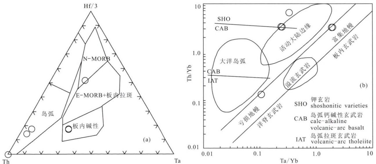
图 10 秦皇岛石门寨蓝旗组火山岩 Th—Hf/3—Ta(a)(据 Wood et al., 1979)和
