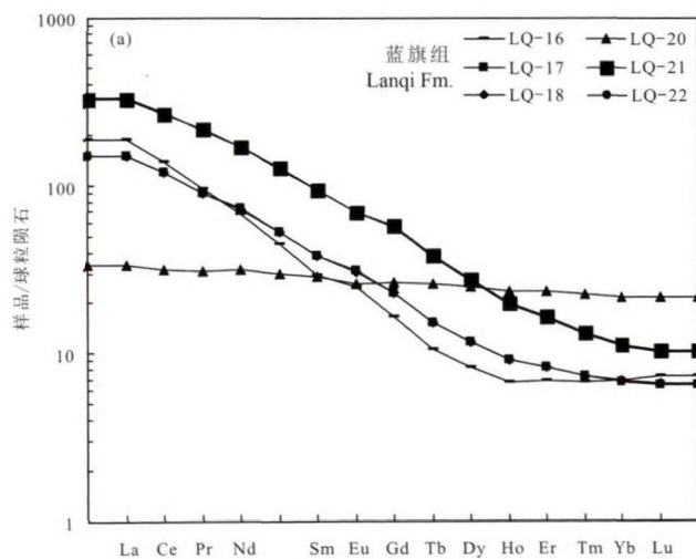
图 8 秦皇岛石门寨蓝旗组(a)和孙家梁组(b)火山岩稀土元素配分曲线模式
