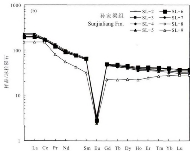
图 8 秦皇岛石门寨蓝旗组(a)和孙家梁组(b)火山岩稀土元素配分曲线模式
