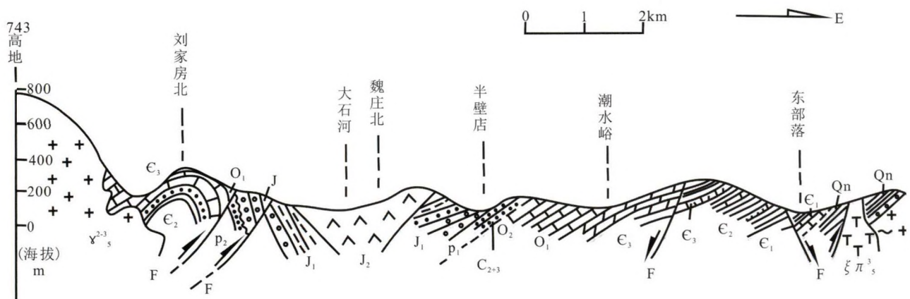
图2 河北秦皇岛柳江盆地地区剖面图
