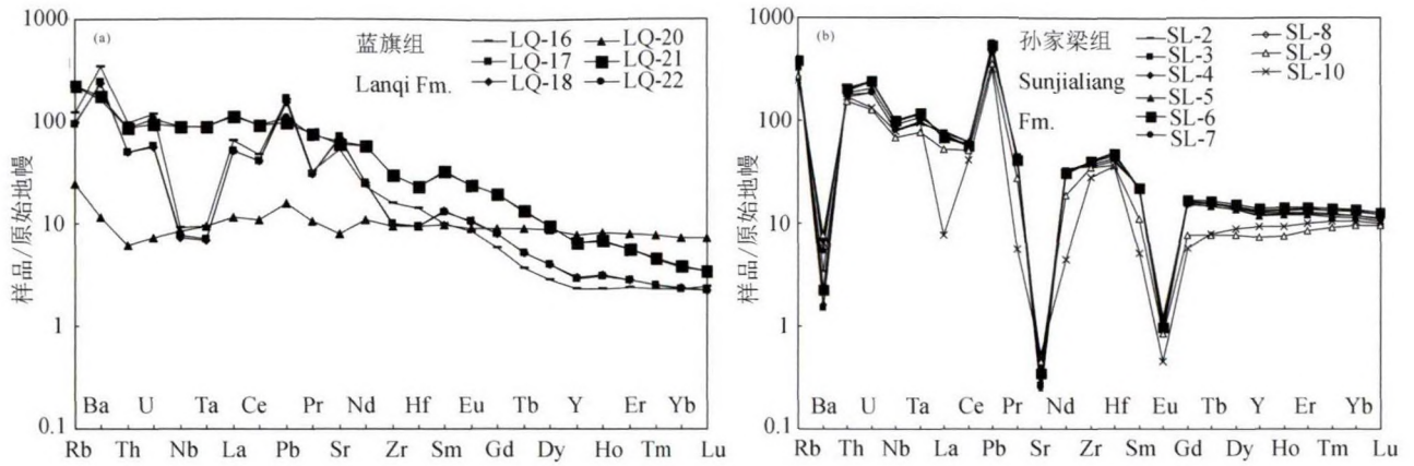
图9 秦皇岛石门寨蓝旗组(a)和孙家梁组(b)火山岩微量元素蛛网图(原始地幔标准值采用 Sun and McDonough, 1989)
