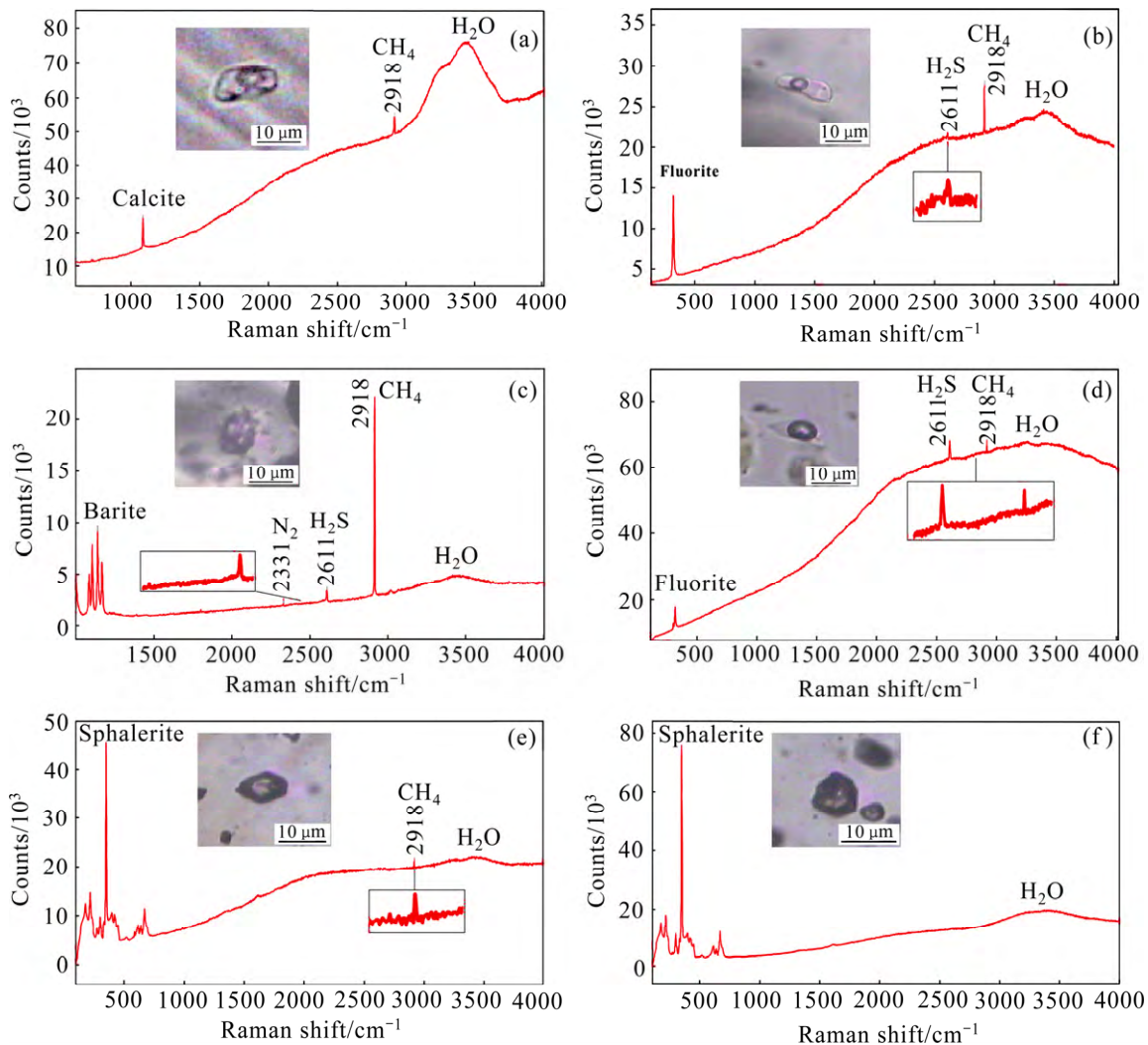
图 8 花垣土地坪铅锌矿床流体包裹体激光拉曼图谱：(a) 阶段方解石中 Ia 型流体包裹体；(b) 阶段萤石 Ia 型流体包裹体；(c) 阶段重晶石中 Ia 型流体包裹体；(d) 阶段萤石 Ib 型流体包裹体；(e) 阶段闪锌矿中 Ia 型流体包裹体；(f) 阶段闪锌矿中 Ia 型流体包裹体
