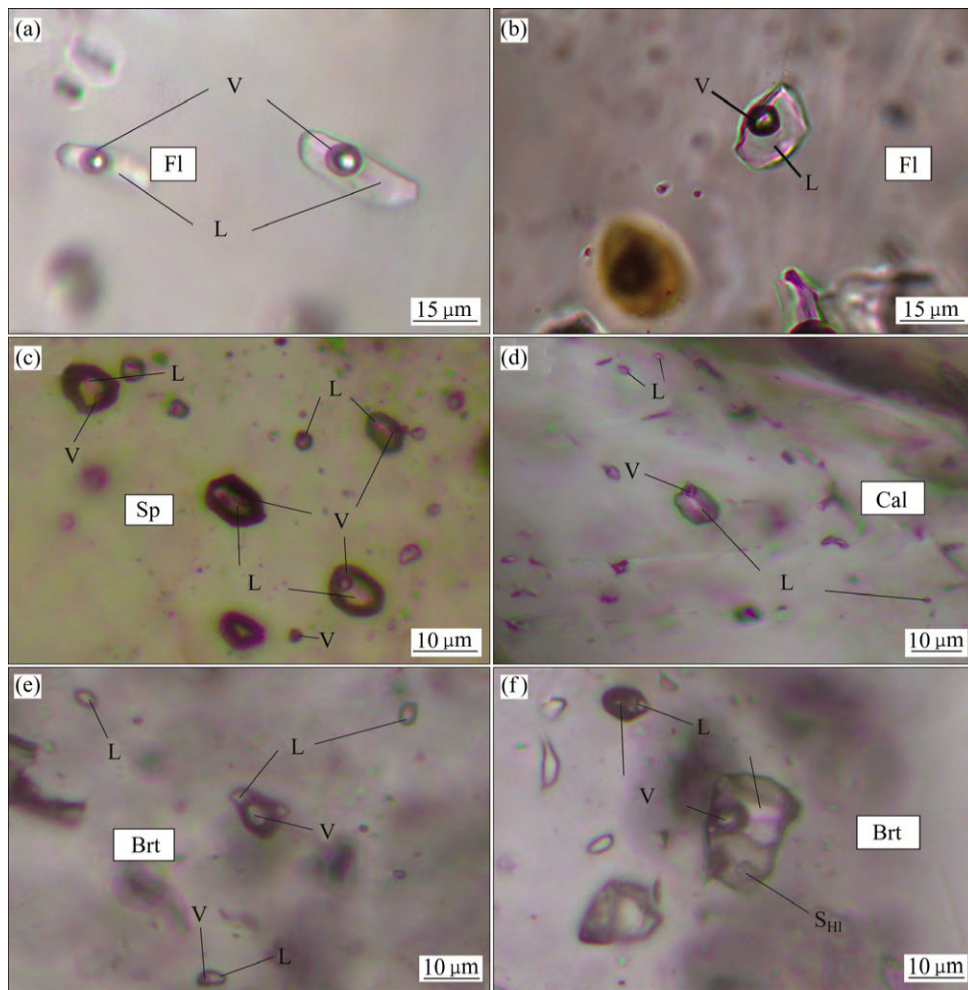
图 6 土地坪铅锌矿床流体包裹体显微照片：(a) 阶段萤石 Ia 型包裹体；(b) 阶段萤石 Ia 型包裹体与黄色有机质伴生；(c) 阶段闪锌矿 Ia 型、与型包裹体；(d) 阶段方解石 Ia 型、型包裹体；(e) 阶段重晶石 Ib 型与型包裹体；(f) 阶段重晶石 Ia 型与型含石盐子晶包裹体伴生；L—液相；V—气相；S—固相；Cal—方解石；Brt—重晶石；FI—萤石；Sp—闪锌矿；HI—石盐
