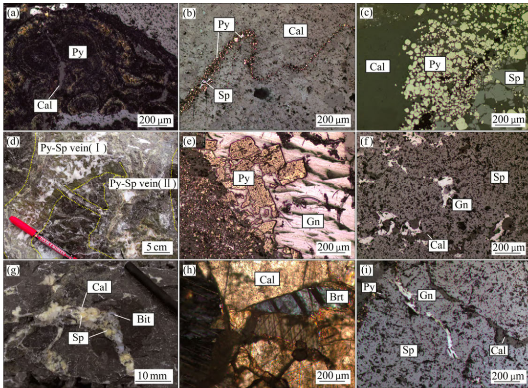
图 5 土地坪铅锌矿床典型矿石结构构造照片：(a) 胶状黄铁矿(-)；(b) 细粒黄铁矿、闪锌矿充填压溶缝合线(-)；(c) 球粒状黄铁矿与半自形闪锌矿共生(-)；(d) 阶段对称的黄铁矿-方铅矿-闪锌矿脉交切 阶段黄铁矿-闪锌矿脉；(e) 立方体晶形黄铁矿被粗粒方铅矿交代呈骸晶结构(-)；(f) 方铅矿交代闪锌矿呈港湾状 (-)；(g) 浅黄色闪锌矿与花斑状方解石、固体沥青共生；(h) 锥状重晶石充填方解石晶隙(+); (i) 细脉状方铅矿充填闪锌矿裂隙(-)；Sp—闪锌矿；Gn—方铅矿；Py—黄铁矿；Cal—方解石；Bit—沥青；Brt—重晶石
