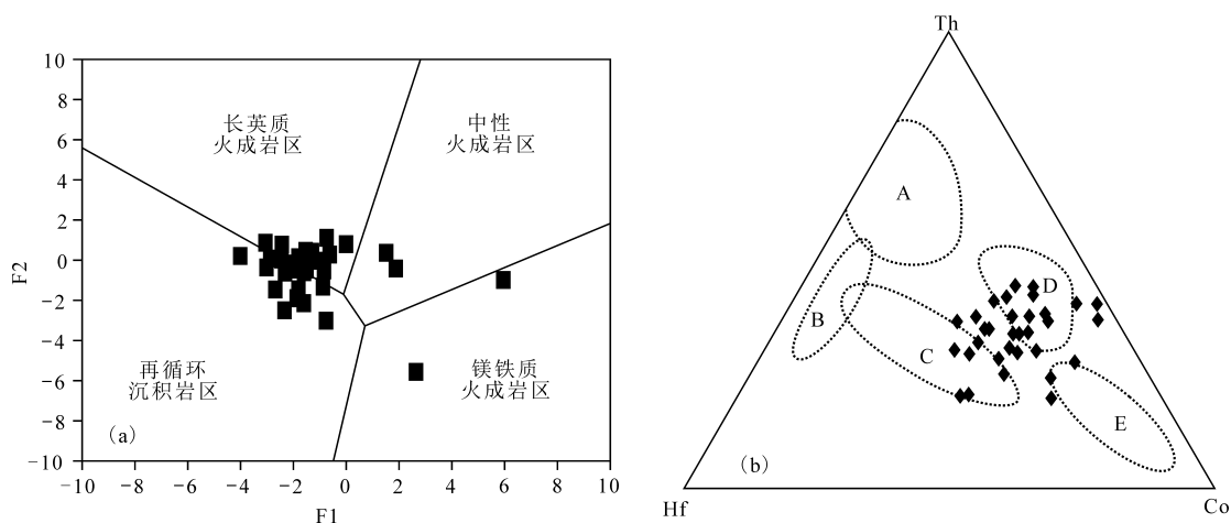
图 6 扶杨油层沉积岩物源判别图
