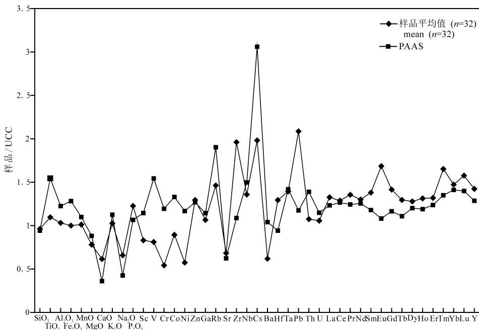
图 3 扶杨油层沉积岩的主要元素与微量元素平均值 UCC 标准化配分图
