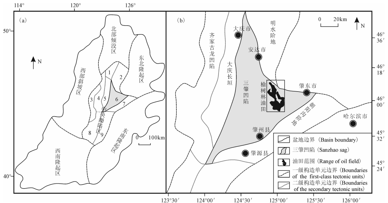
图1 松辽盆地构造分区图(a)及榆树林油田区域位置图(b)(据谭保祥等,1995;刘媛,2010 改编)
