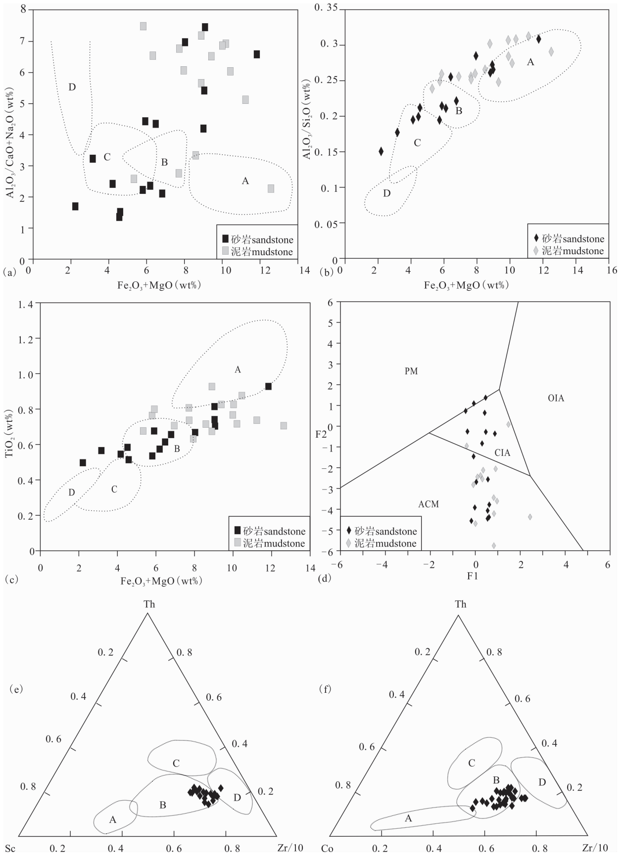
图7 扶杨油层沉积岩构造背景判别图
