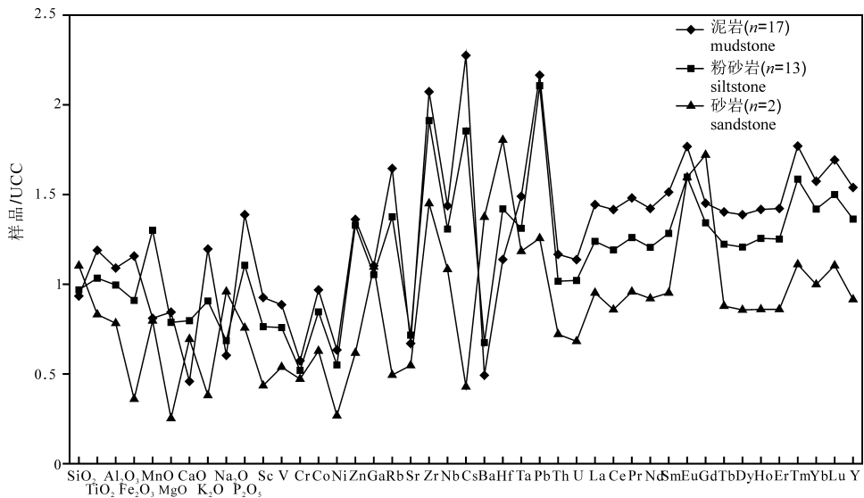
图4 扶杨油层泥岩—粉砂岩—砂岩主微量元素平均值 UCC 标准化配分图
