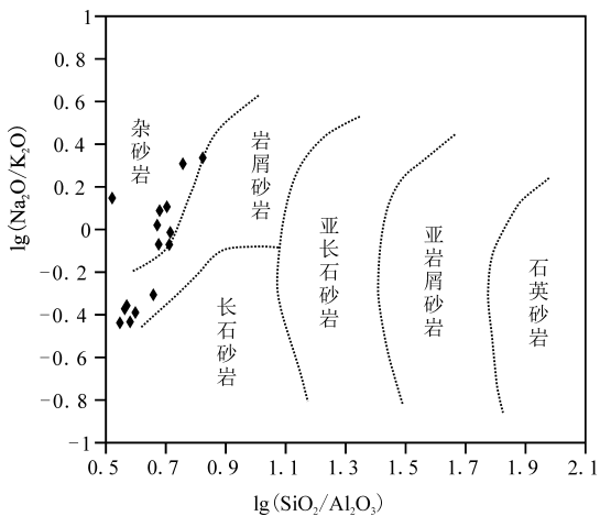
图5 扶杨油层砂岩类型主元素判别图 (据 Pettijhon et al., 1972)
