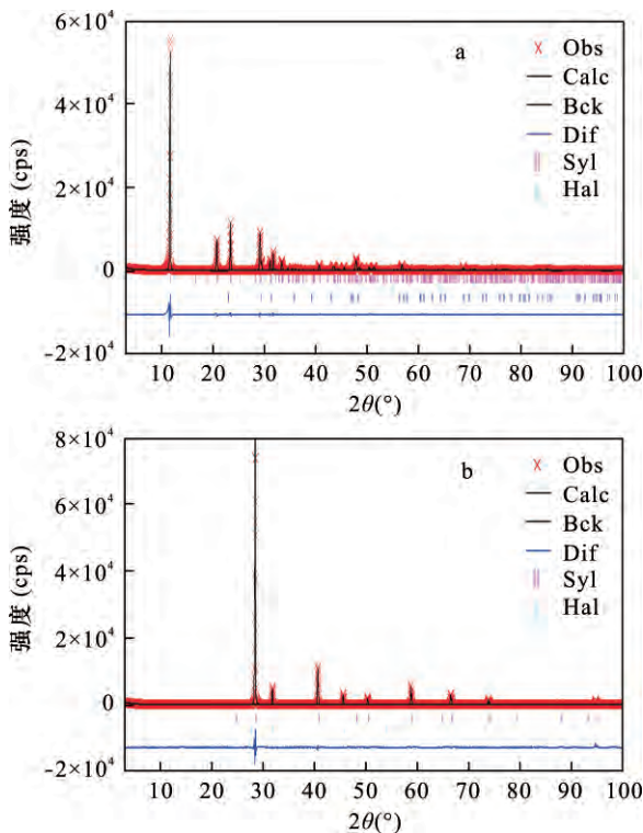
a—石膏样品; b—钾盐样品。Obs—实测数据; Calc—计算数据; Bck—背景曲线; Dif—差值曲线; Syl—钾盐; Hal—石盐; Cal—方解石。
