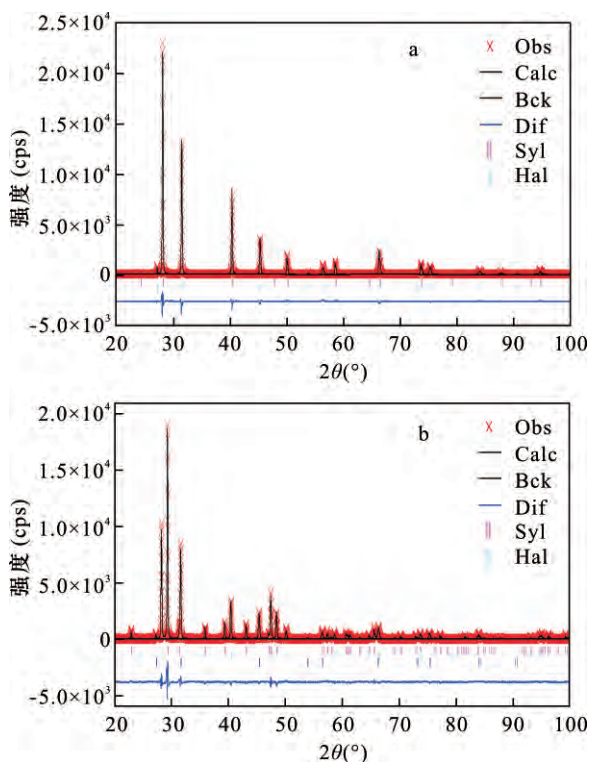
a—SH46 样品; b—SHC226 样品。Obs—实测数据; Calc—计算数据; Bck—背景曲线; Dif—差值曲线; Syl—氯化钾; Hal—氯化钠; Cal—碳酸钙。
