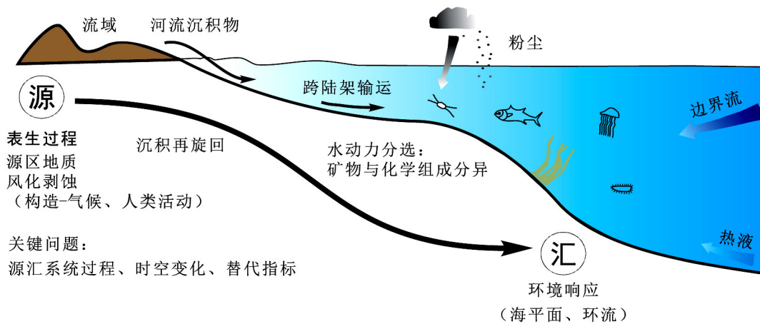
图1 东亚大陆边缘沉积物从源到汇过程研究的特色与复杂性
