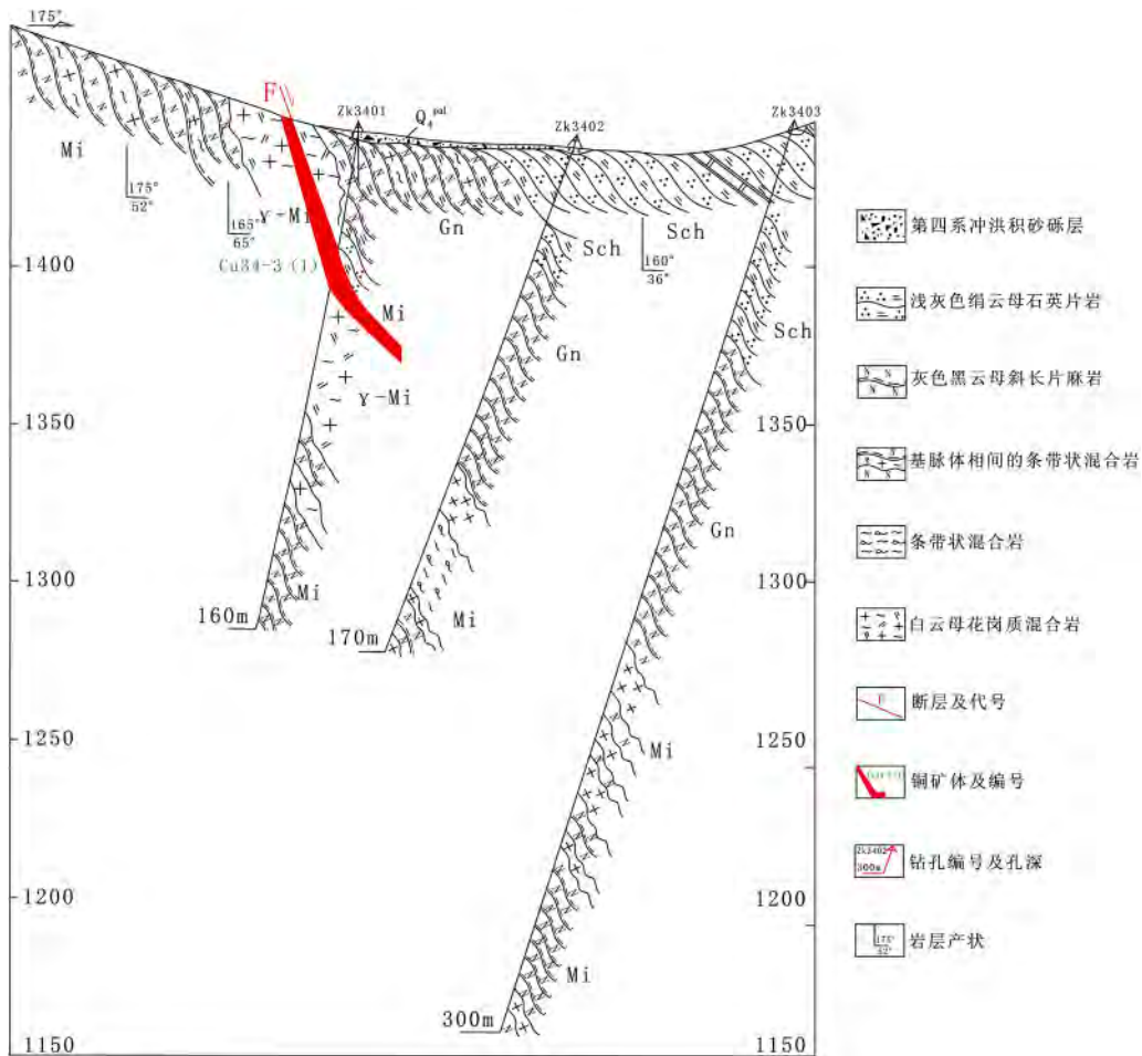
图 2 包尔图铜矿区 34 号勘探线剖面图
