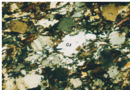
黑云斜长片麻岩正交偏光,放大 25 倍
