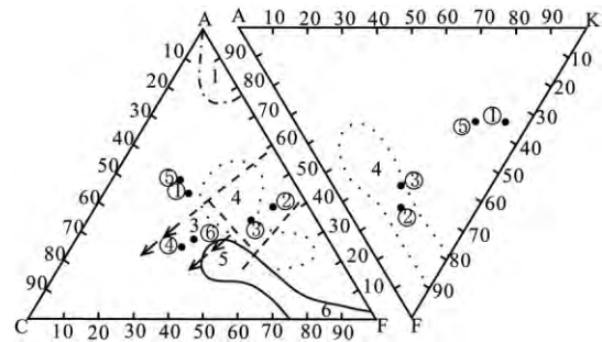
图6 ACF和 A'KF 图解
