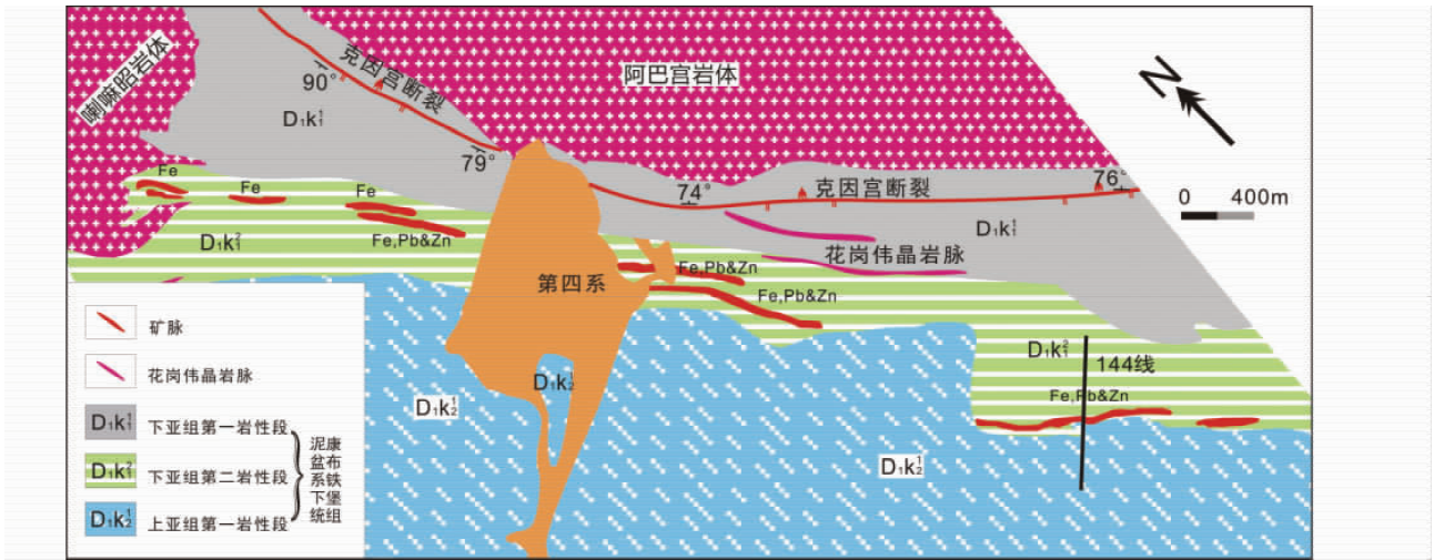
图2 塔拉特铁铅锌矿床地质简图(据袁建江等, 2011 修改)
