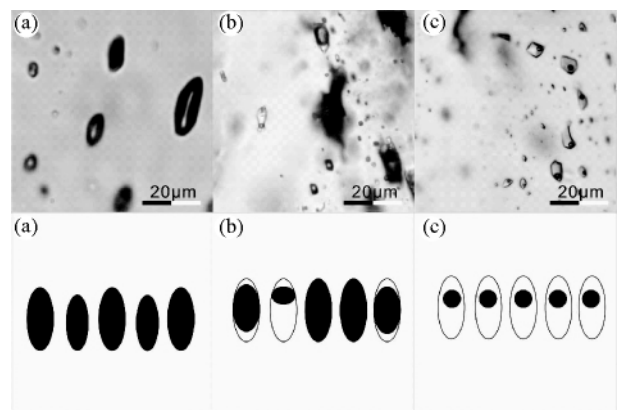
图10 塔拉特铁铅锌矿床流体演化特征
