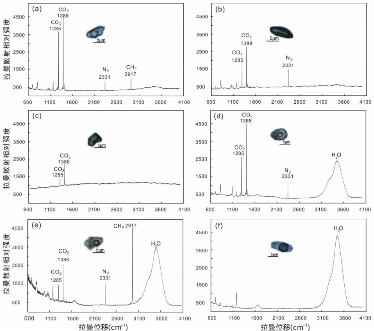
图7 塔拉特铁铅锌矿床流体包裹体激光拉曼谱图
