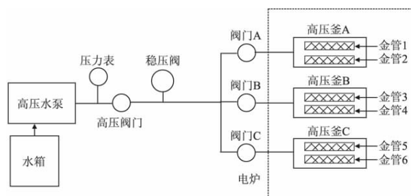
图1 黄金管—高压釜限定体系装置
