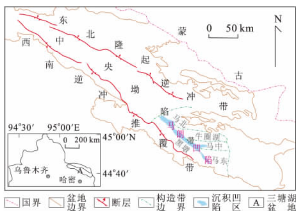
图1 马朗凹陷区域位置及构造单元划分
