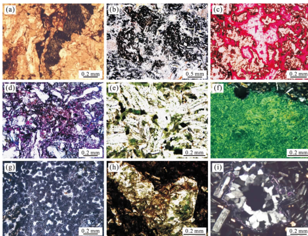
图4 马朗凹陷卡拉岗组火山岩典型矿物特征
