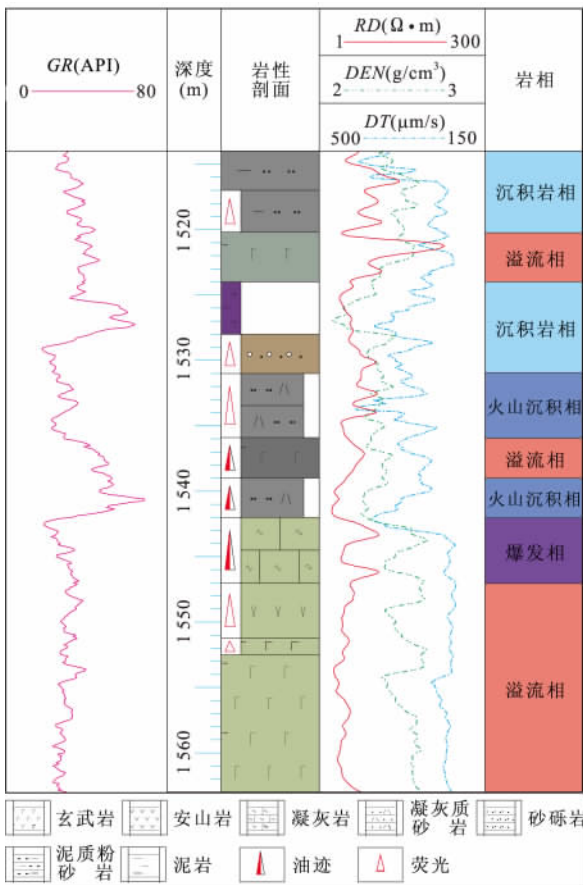
图 2 马朗凹陷卡拉岗组火山岩测井相分析
