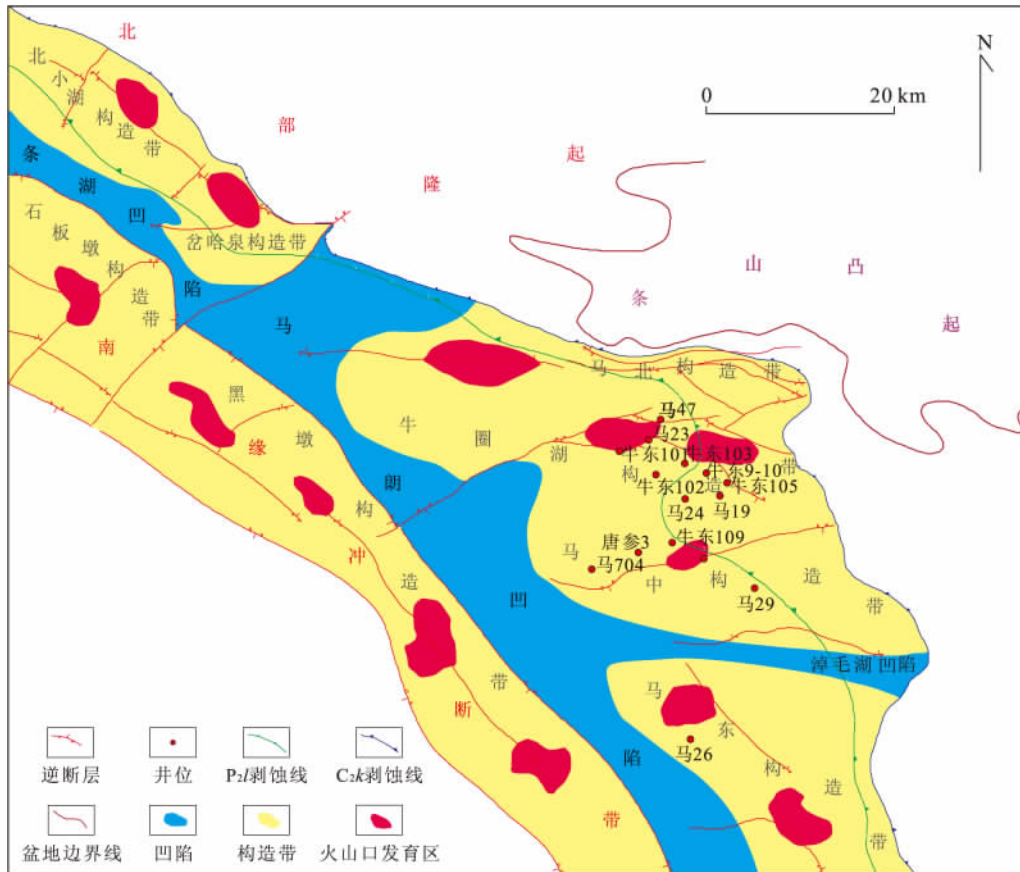
图 3 马朗凹陷石炭系卡拉岗组火山分布与断裂关系
