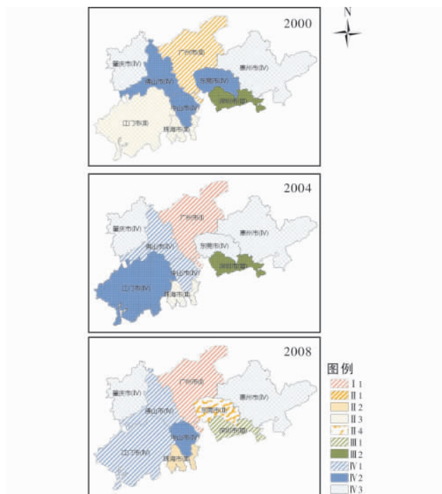
图 3 2000、2004、2008 年城市自然灾害应对能力类型演变分布图
