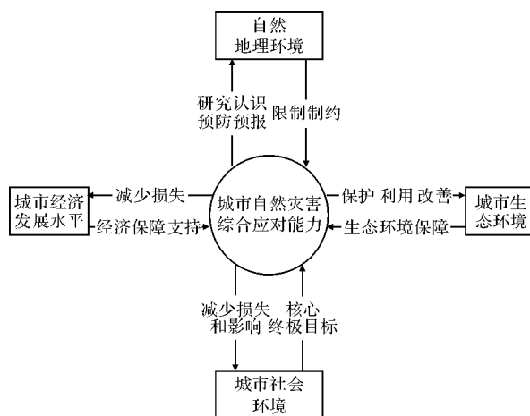
图1 城市灾害应对能力与城市系统关系
