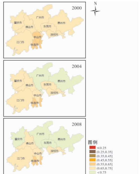
图 2 2000、2004、2008 年城市自然灾害应对能力分类变化图
