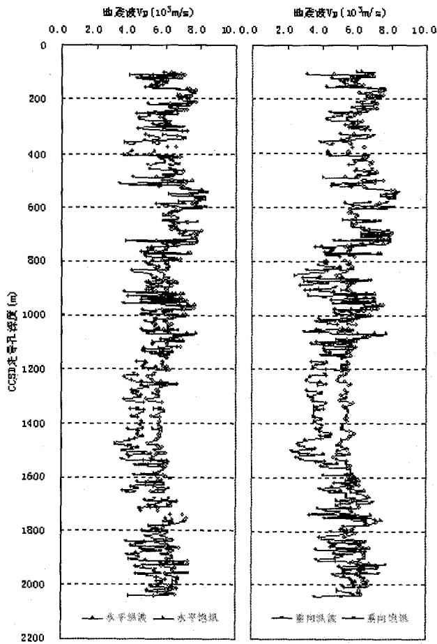
图2 CCSD主孔2000米地震纵波速度在饱水前后随深度变化剖面图
