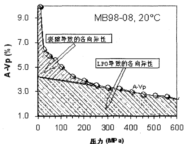
图 9 东海地表榴辉岩地震波各向异性与岩石微裂隙和 LPO 之间的关系(样品 MB98-08)
