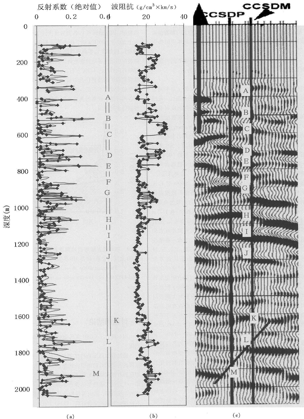
图8 CCSD 主孔 2000 米岩石的反射系数(a)、波阻抗(b)与地球物理反射剖面(c, 据杨文采等,2002)对照图
